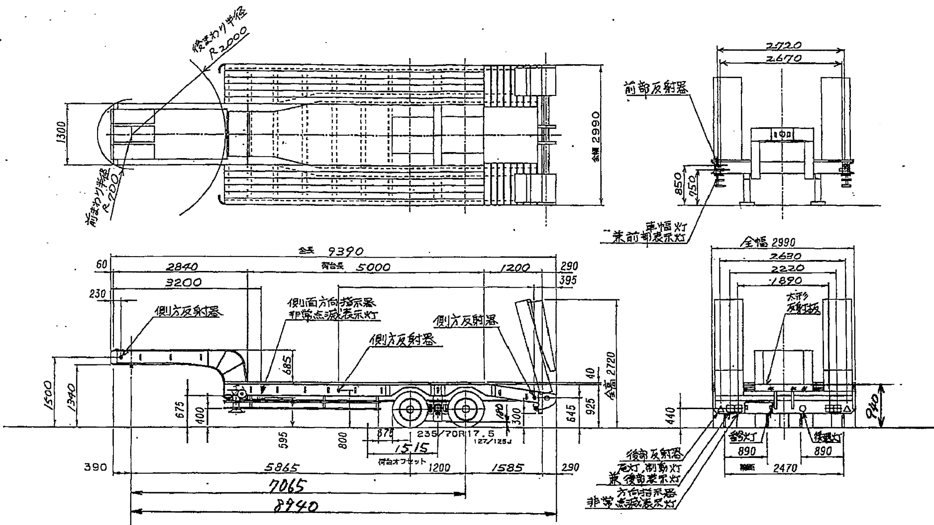
トレーラーモービル PLR430AK型 外観四面図
